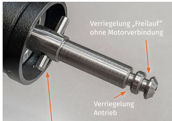
Antriebsstift: Motor greift in die Adapterplatte des Rades.
